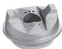
Ghiera/ Lock nut
